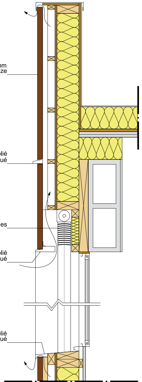
Coupe verticale
