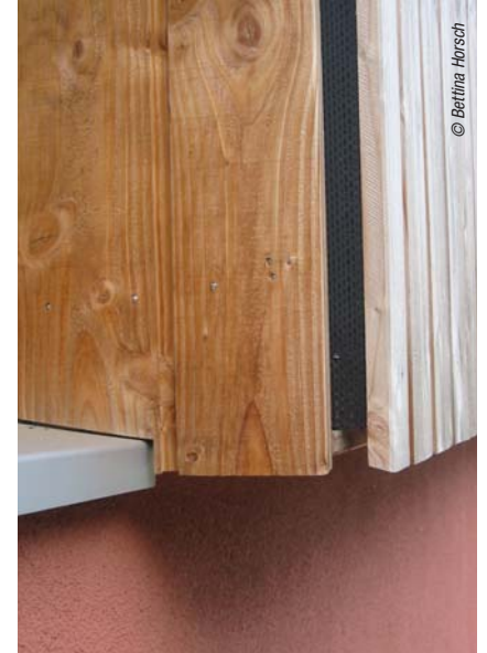
Ici, le joint vertical entre les lames de la façade et celles de l'encadrement de la fenêtre est ouvert, avec une grille anti-rongeur située derrière.
