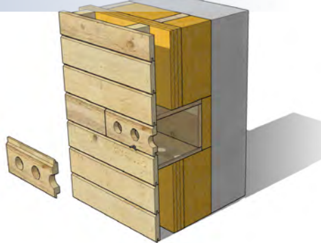
Intégration d'un nichoir dans un bardage
