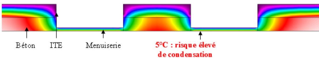
Figure 8 - Illustration de ponts thermiques au niveau des menuiseries. Modélisation sous THERM d'une isolation extérieure avec menuiseries au nu intérieur sans retour d'isolant en tableau : les points froids sont tels qu'ils provoquent un sentiment d'inconfort (paroi froide) et un risque élevé de condensation. (Source : Enertech)
