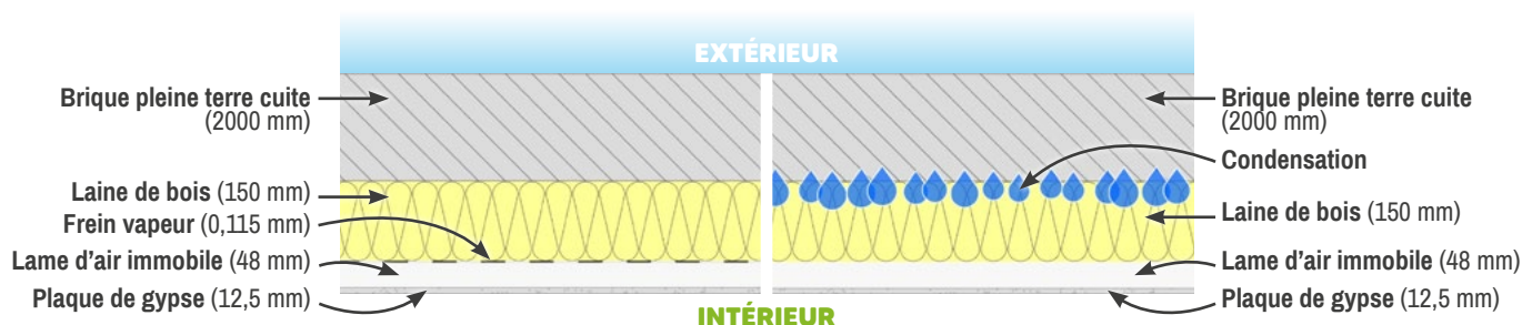
Figure 23 - Paroi brique rénovée avec une solution d'ITI avec (gauche) et sans (droite) mise en œuvre d'un frein-vapeur - Source : ubakus.com / CODEM
