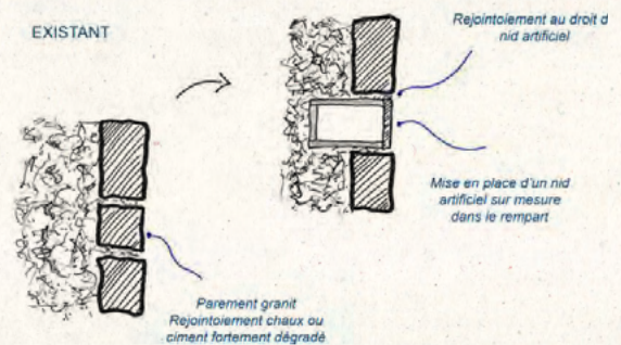
Dessins présentant les différents dispositifs de nichoirs mobilisés dans le projet de restauration des remparts de Guérande (44) : maintien de cavités existantes, création de nids artificiels... | © Perrot & Richard, architectes
